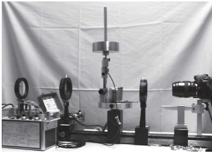
圖三：實驗所採用之光彈組合。
